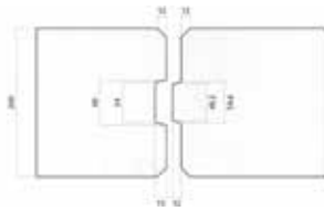
[TG 200T 일반형]
