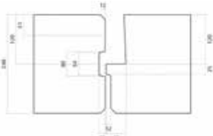
[TGG 240T 철근보강형]
