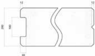
[GV 200T 수직벽체형]
